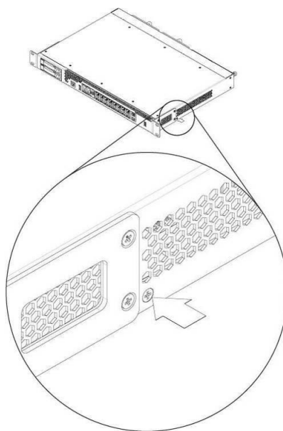
Рисунок 19 — Сборка в корпус
