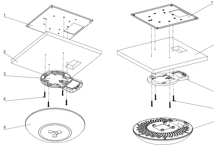
Рисунок 9 – Монтаж устройства на фальшпотолок
