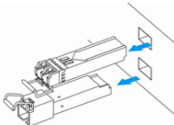
Рисунок 82 – Извлечение SFP-трансиверов
