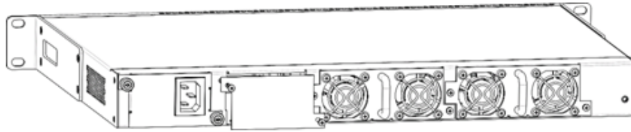
Рисунок 78 – Установка заглушки
