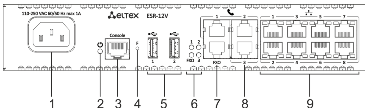
Рисунок 55 – Передняя панель ESR-12V
