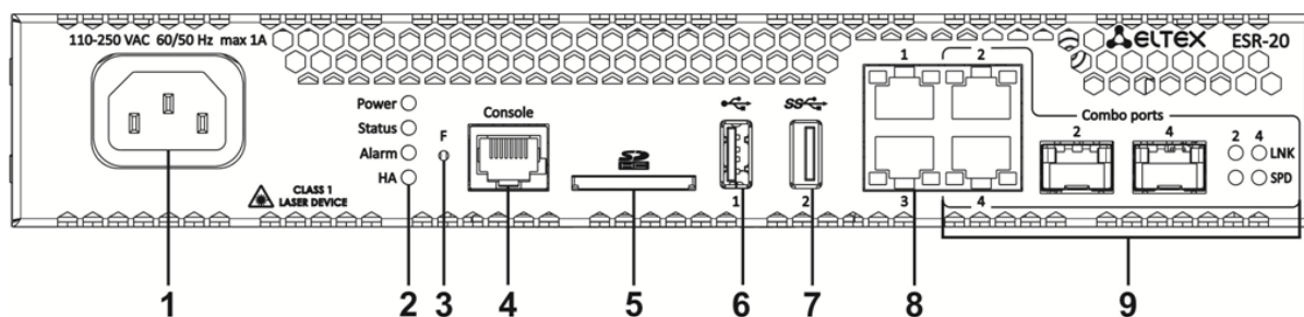
Рисунок 37 – Передняя панель ESR-20
