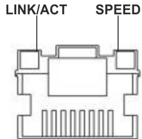
Рисунок 62 – Расположение индикаторов разъема RJ-45
