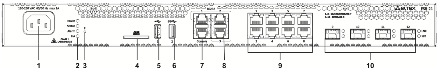
Рисунок 32 – Передняя панель ESR-21
