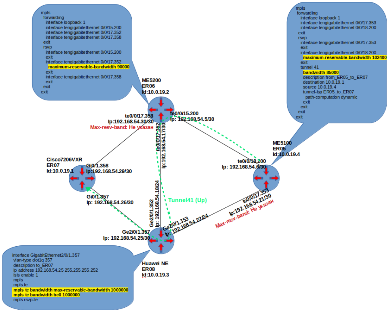
Figure 1. Пример 1: Конфигурация TE-туннеля с требованием резервирования полосы пропускания 85 Mbps.
