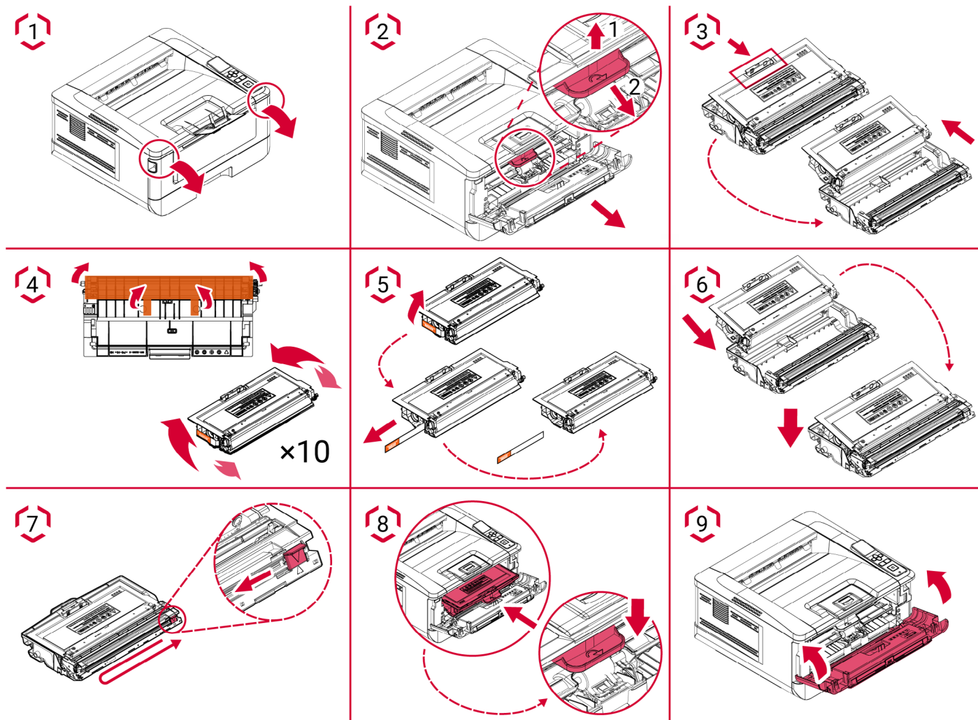
Рисунок 35 – Замена картриджа
