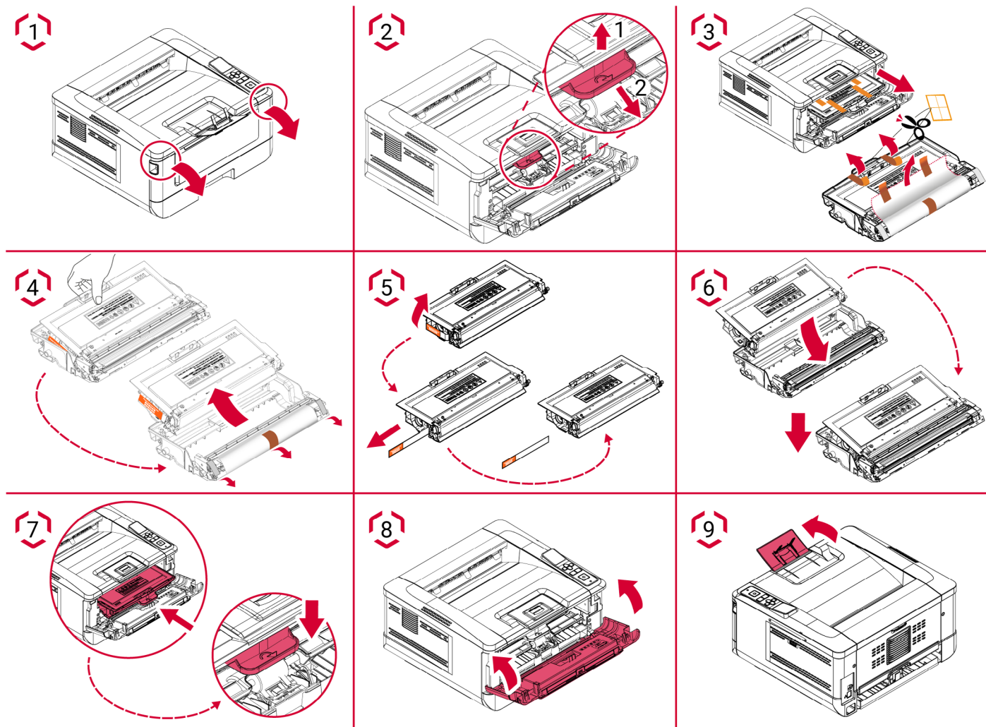
Рисунок 4 – Подготовка тонер-картриджа
