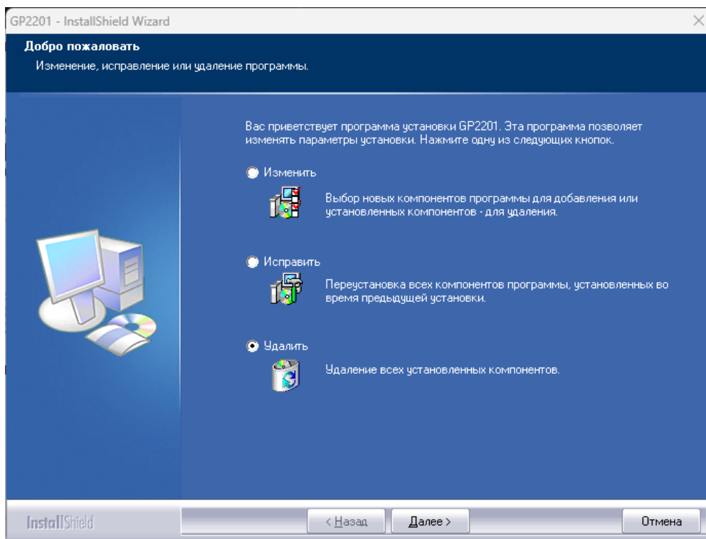
Рисунок 21 – Удаление драйверов
