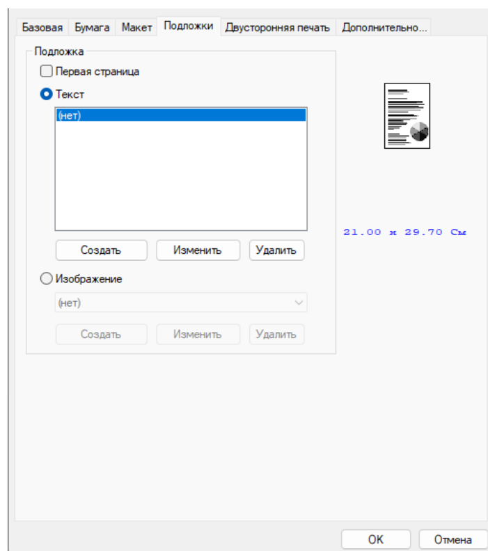
Рисунок 27 – Вкладка «Подложки»
