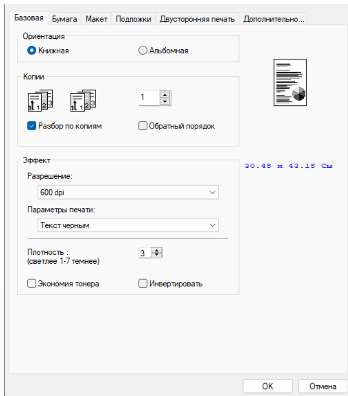
Рисунок 23 – Вкладка «Базовая»
