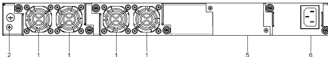
Рисунок 42 — Задняя панель MES3400-24, MES3400I-24, MES3400-48
