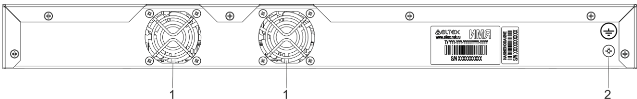
Рисунок 40 – Задняя панель MES2411X
