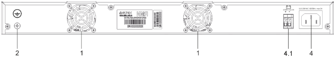
Рисунок 37 – Задняя панель MES2448B
