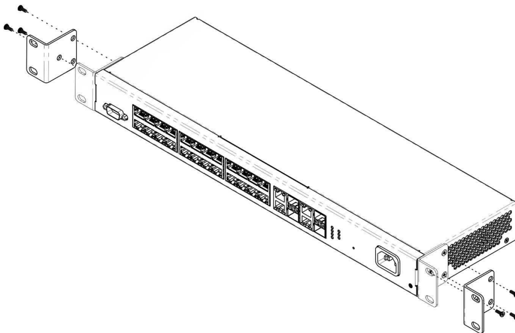
Рисунок 54 – Крепление кронштейнов
