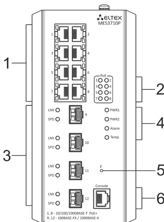
Рисунок 32 – Передняя панель MES3710P
