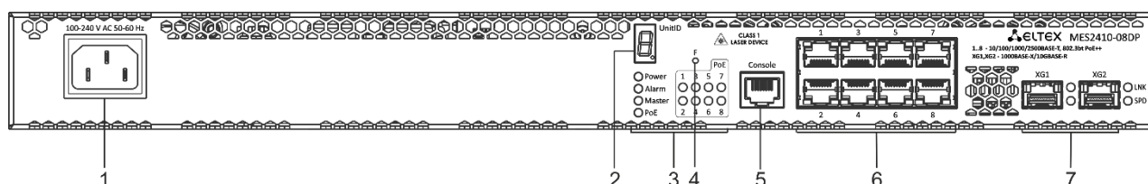
Рисунок 30 – Передняя панель MES2410-08DP
