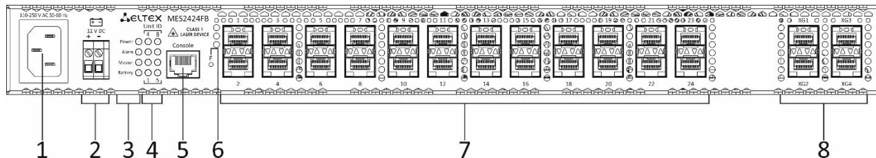
Рисунок 28 — Передняя панель MES2424FB
