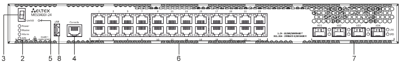
Рисунок 26 – Передняя панель MES3400I-24
