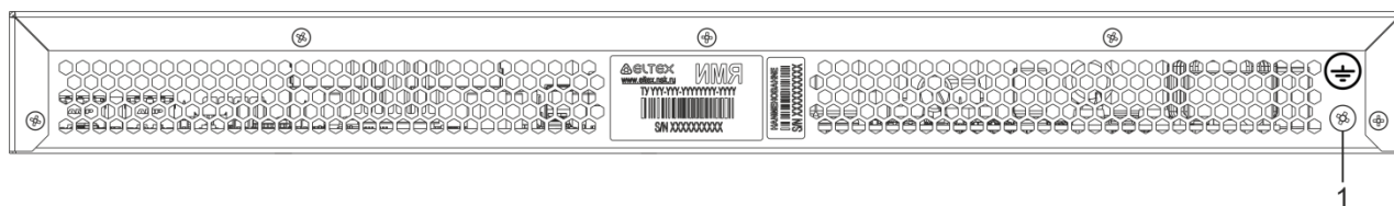
Рисунок 33 – Задняя панель MES1428, MES2428, MES2428T, MES2428B, MES2408IP DC1, MES2408P, MES2424 и MES2424B
