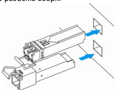
Рисунок 57 – Установка SFP-трансиверов
