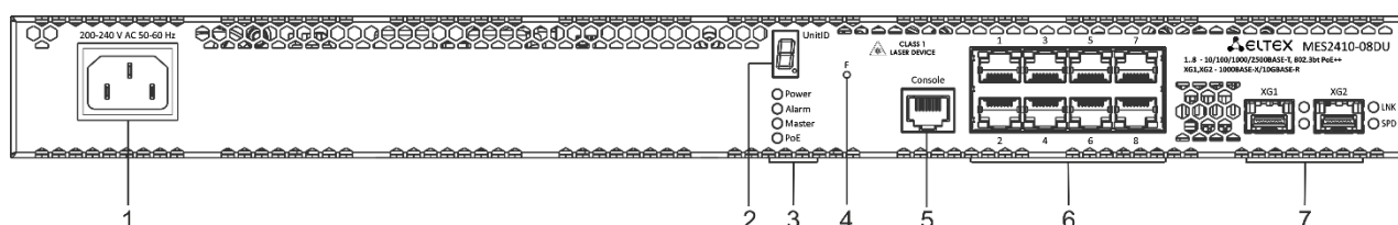
Рисунок 31 – Передняя панель MES2410-08DU
