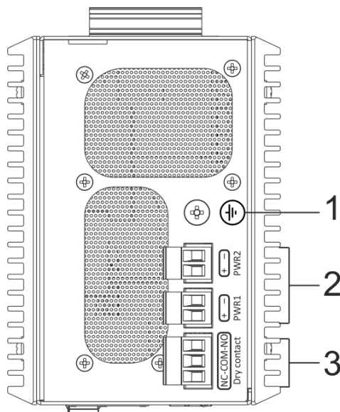
Рисунок 45 — Верхняя панель MES3710P
