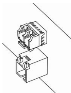
Рисунок 58 – Установленные SFP-трансиверы
