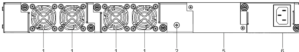
Рисунок 43 — Задняя панель MES3400-24F
