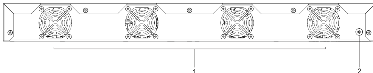
Рисунок 43 — Задняя панель MES3400-24F
