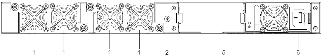
Рисунок 39 – Задняя панель MES2420-48P
