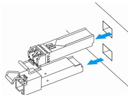
Рисунок 60 – Извлечение SFP-трансиверов
