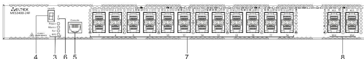
Рисунок 29 — Передняя панель MES3400-24F
