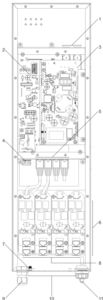
Рисунок 48 – Основные компоненты и разъемы MES3708P
