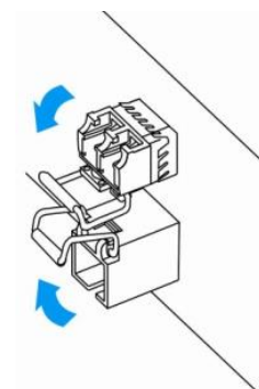
Рисунок 59 – Открытие защелки SFP-трансиверов
