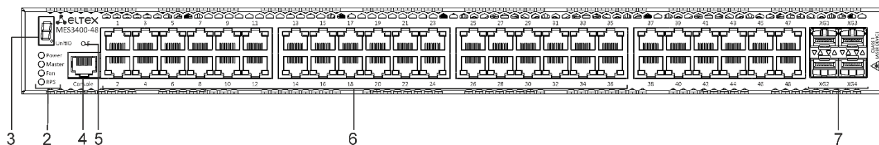
Рисунок 27 – Передняя панель MES3400-48
