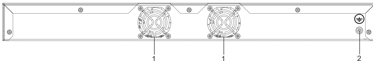
Рисунок 35 – Задняя панель MES2424P, MES2428P
