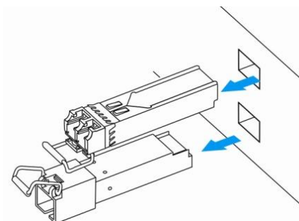
Рисунок 42 – Извлечение SFP-трансиверов
