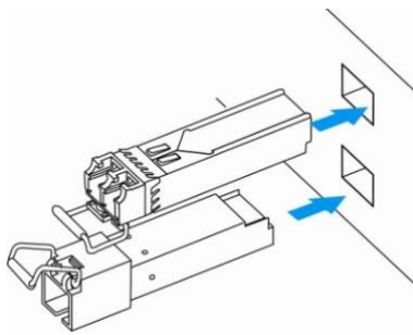
Рисунок 39 – Установка SFP-трансиверов
