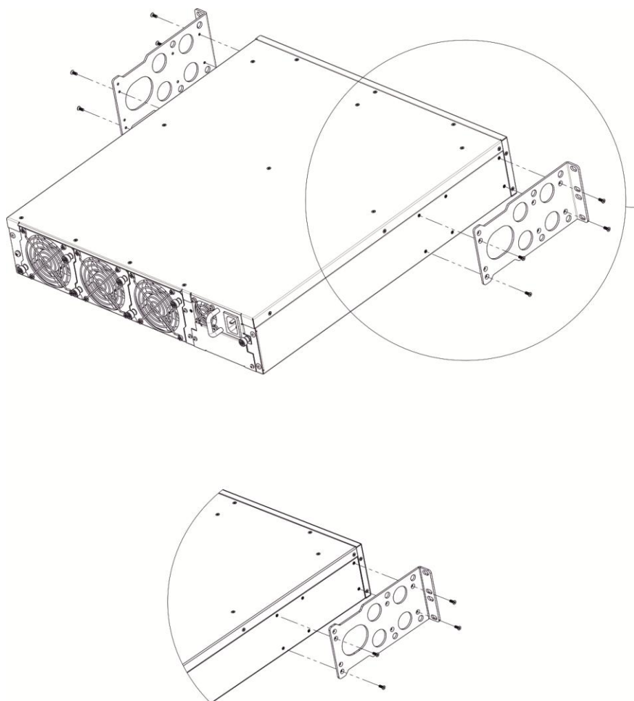
Рисунок 11 – Крепление кронштейнов
