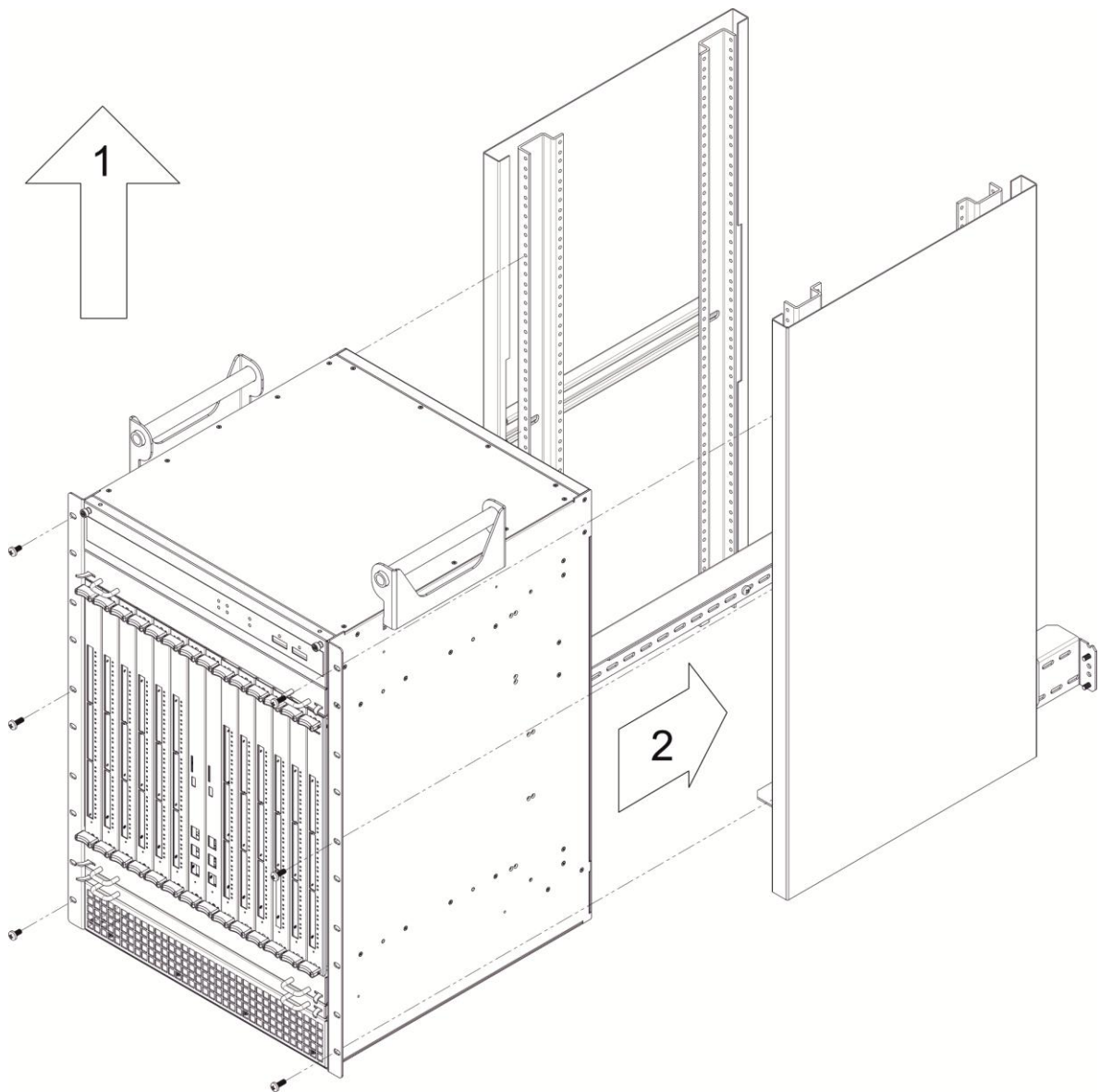
Рисунок 16 – Установка шасси ME5000 в стойку
